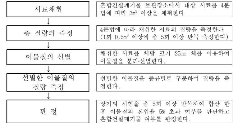
[그림 4] 간편법 2 측정절차(1m 3 -톤백 용기사용)
