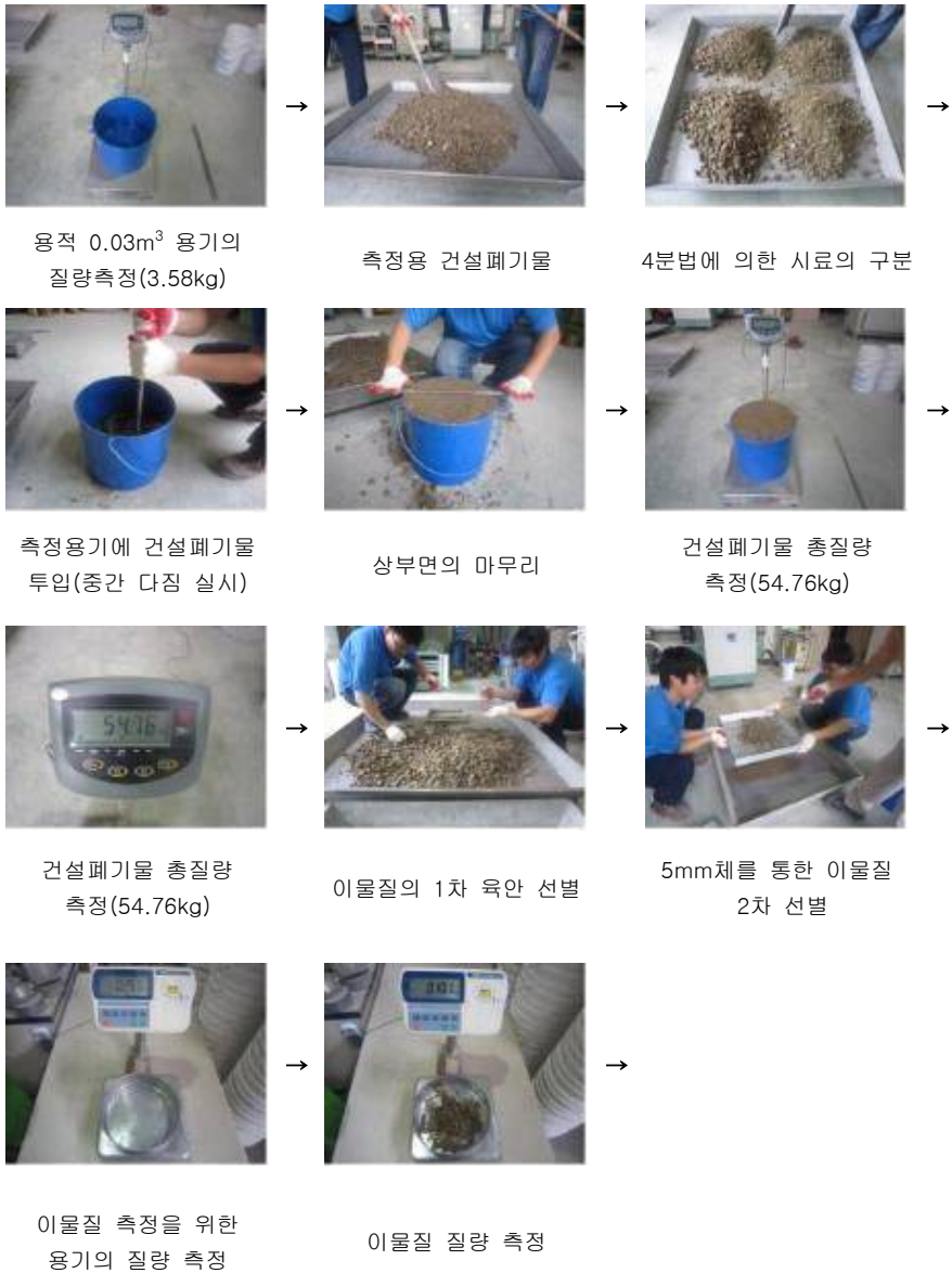
[그림 5] 간편법 1 측정절차(1회 0.03m³, 총 0.15m³ 이상 측정(5회 이상)하여 합산)
