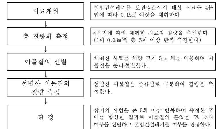
[그림 3] 간편법 1 측정절차(0.03m³ 표준용기 사용)
